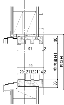
断面図
