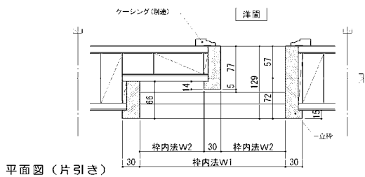
平面図 (片引き)
