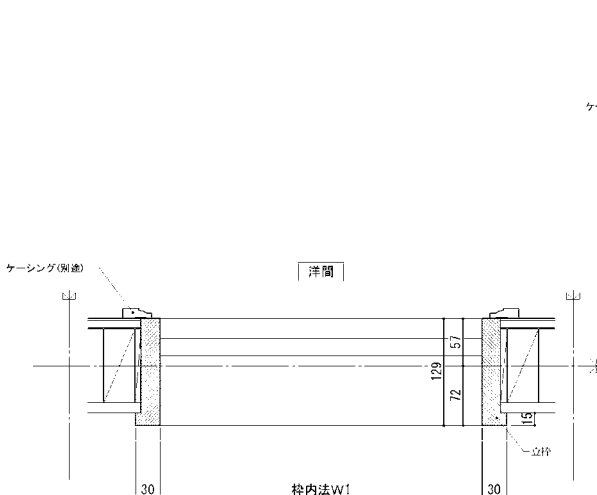
平面図
