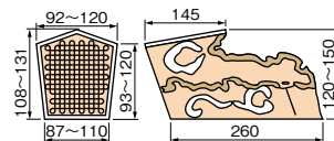
万能隅木
