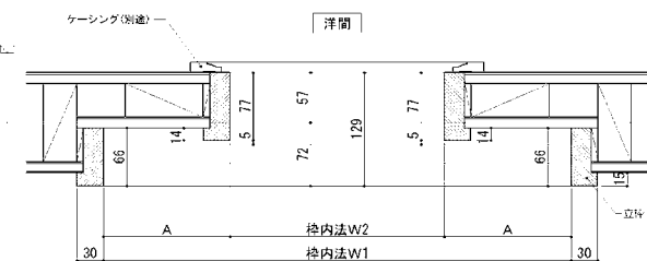
平面図 (引分け)
