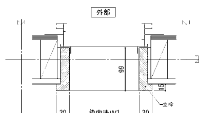
平面図
