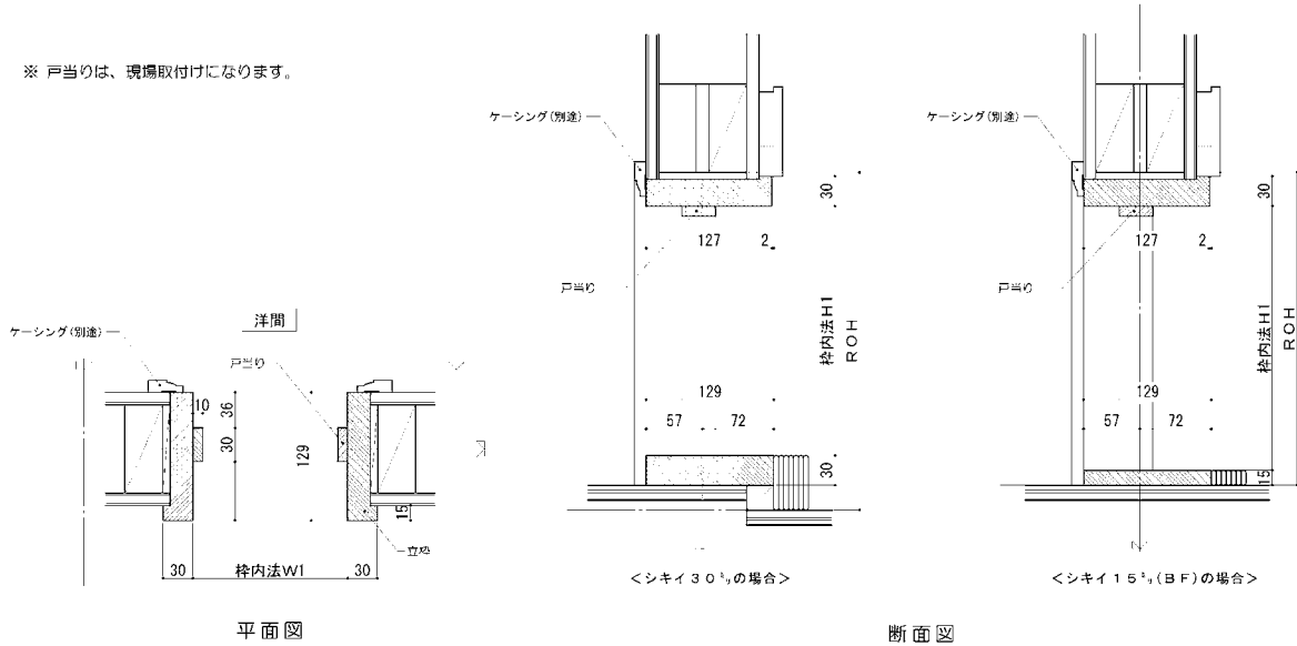
断面図
